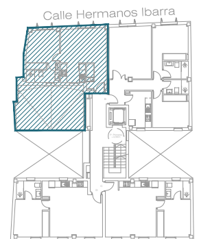
P. 1ª ESCALA 1/100
